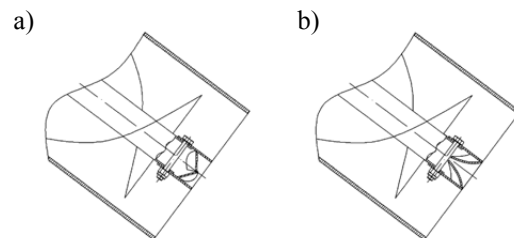
3 pav. Principinė antgalių tvirtinimo schema: trijų menčių (a), dviejų menčių (b)
