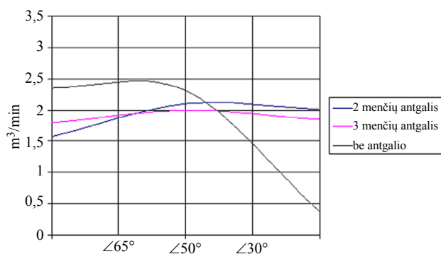
4 pav. Ežektoriaus oro kiekis Fig. 4. Ejected air flow
